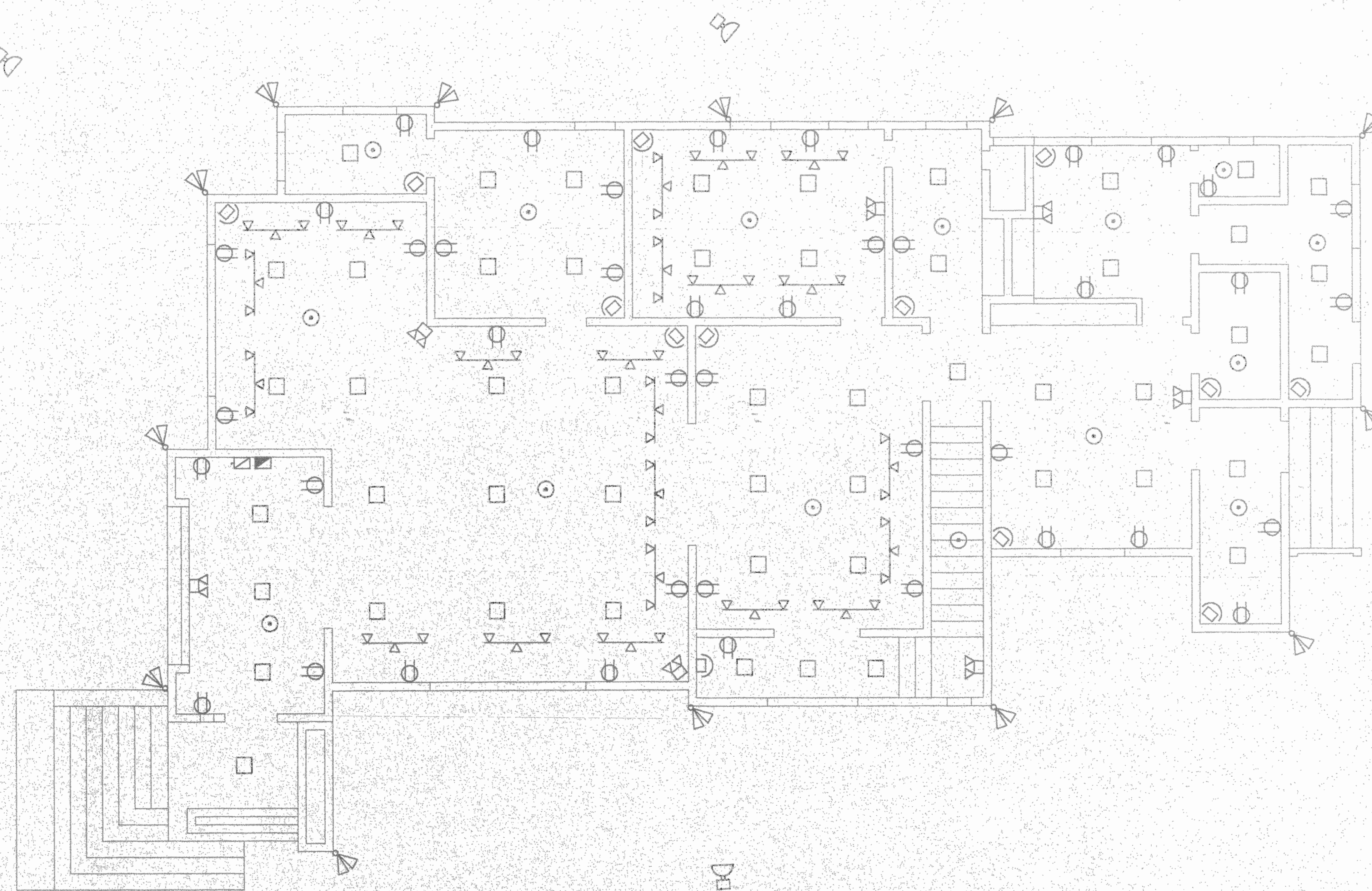
PLANTA DISTRIBUCION ELECTRICA BAJA ESC. 1 : 50
