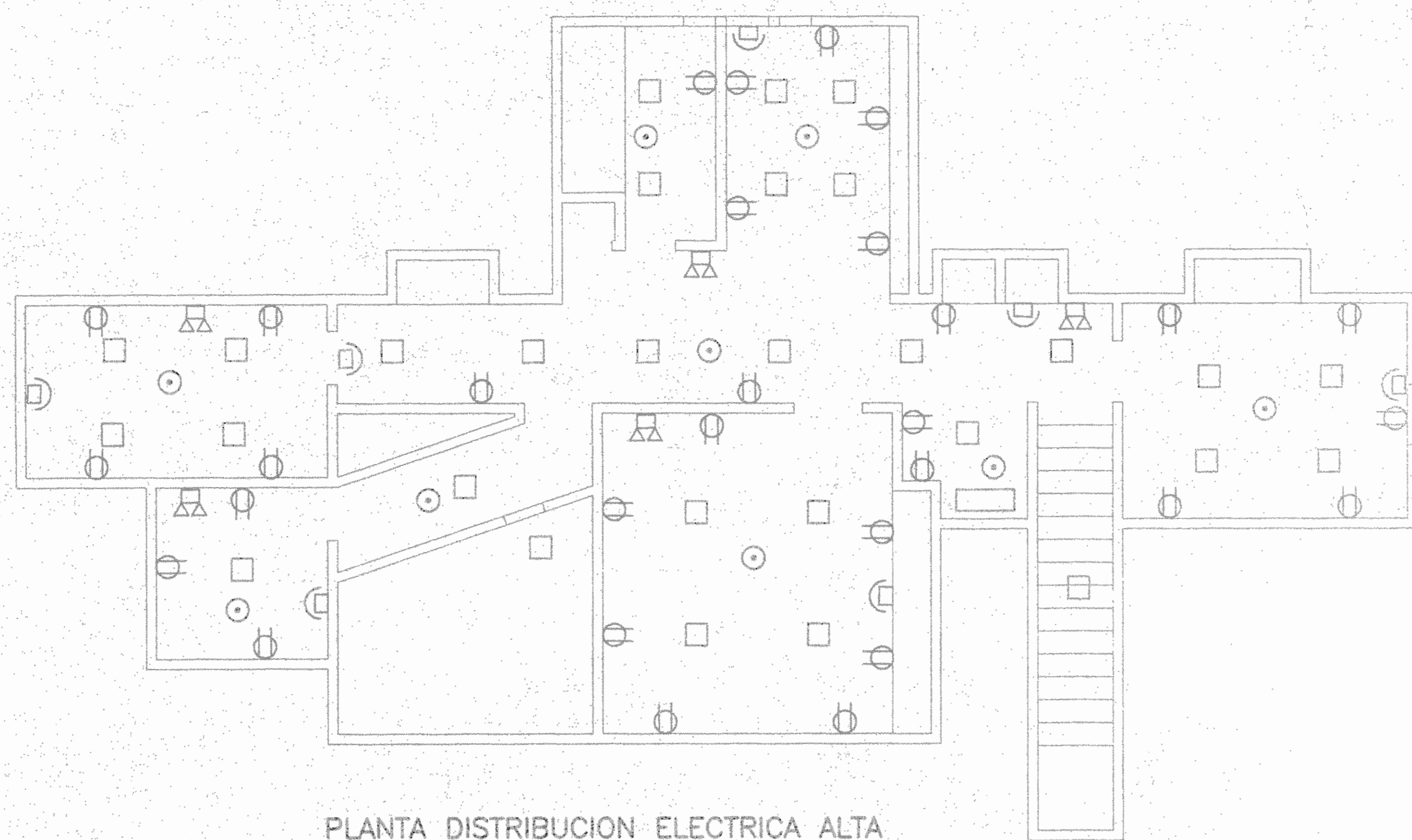
PLANTA DISTRIBUCION ELECTRICA ALTA ESC. 1 : 50
